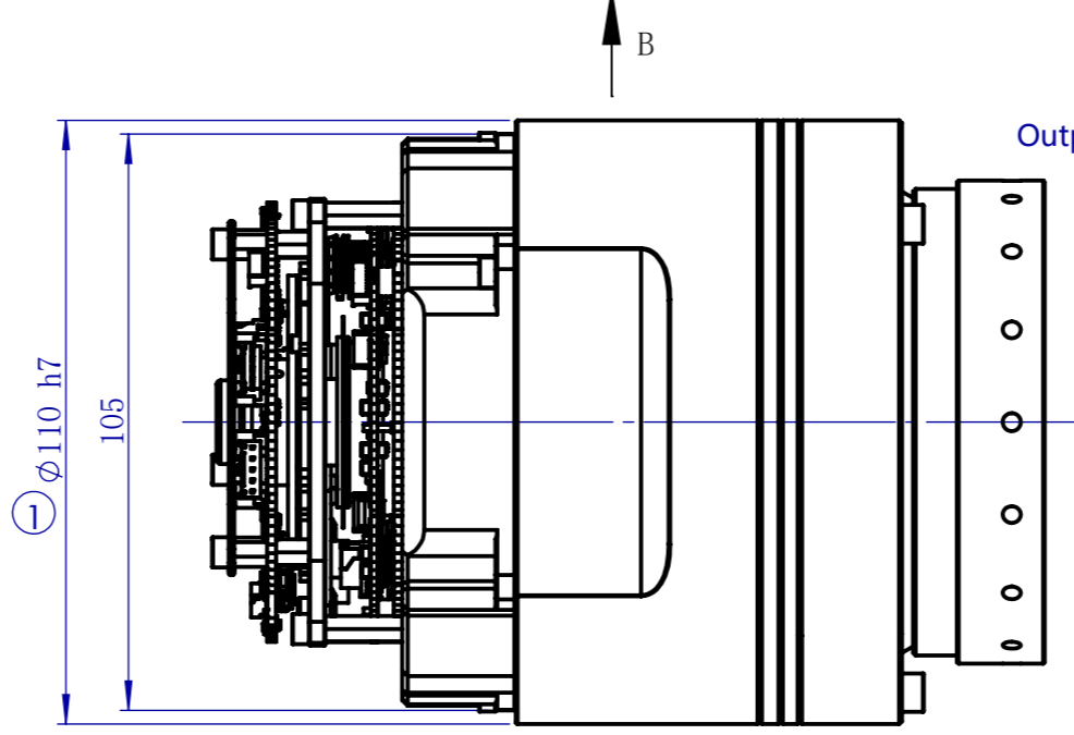
视图 B View B 比例 1 : 1.5 Scale 1:1.5
