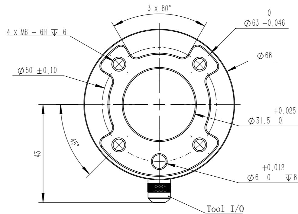
工具法兰 比例 1 : 1
