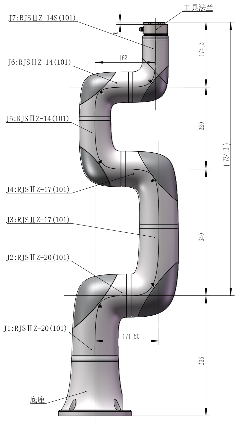
比例 1 : 5
