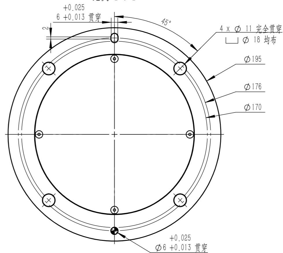
底座 比例 1 : 2
